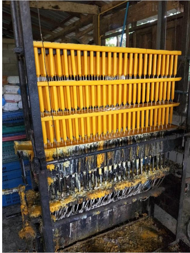
ผลิตตัวเทียนด้วยเครื่องหล่อเทียน
